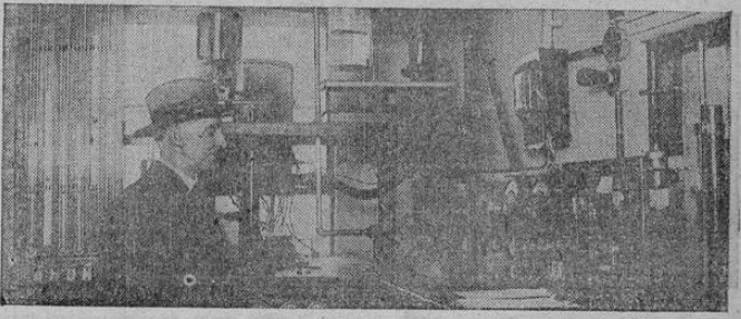
El doctor C. Dickenson es el jefe de la oficina encargada de probar los motores de los aeroplanos fabricados en los Estados Unidos. Aquí se le ve en su cuarto de trabajo, en Arlington, Virginia
